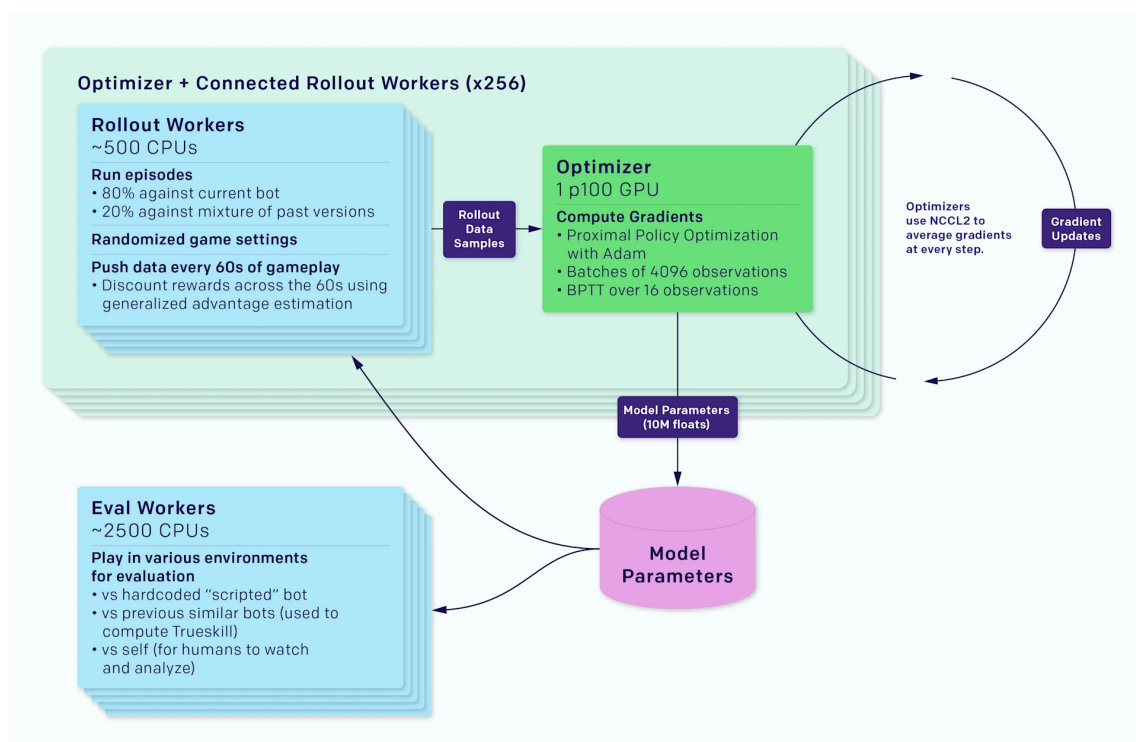
Obrázek 1.6: Architektura tréninkového systému OpenAI Five. Rollout workeři generují data ze zápasů, která jsou následně zpracována optimalizačním modulem využívajícím metodu PPO. Výsledné aktualizace jsou sdíleny napříč instancemi a evaluovány ve specifických herních prostředích.[25]
